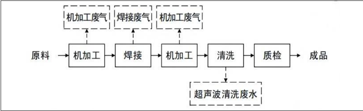
图 4-1 工艺流程图
